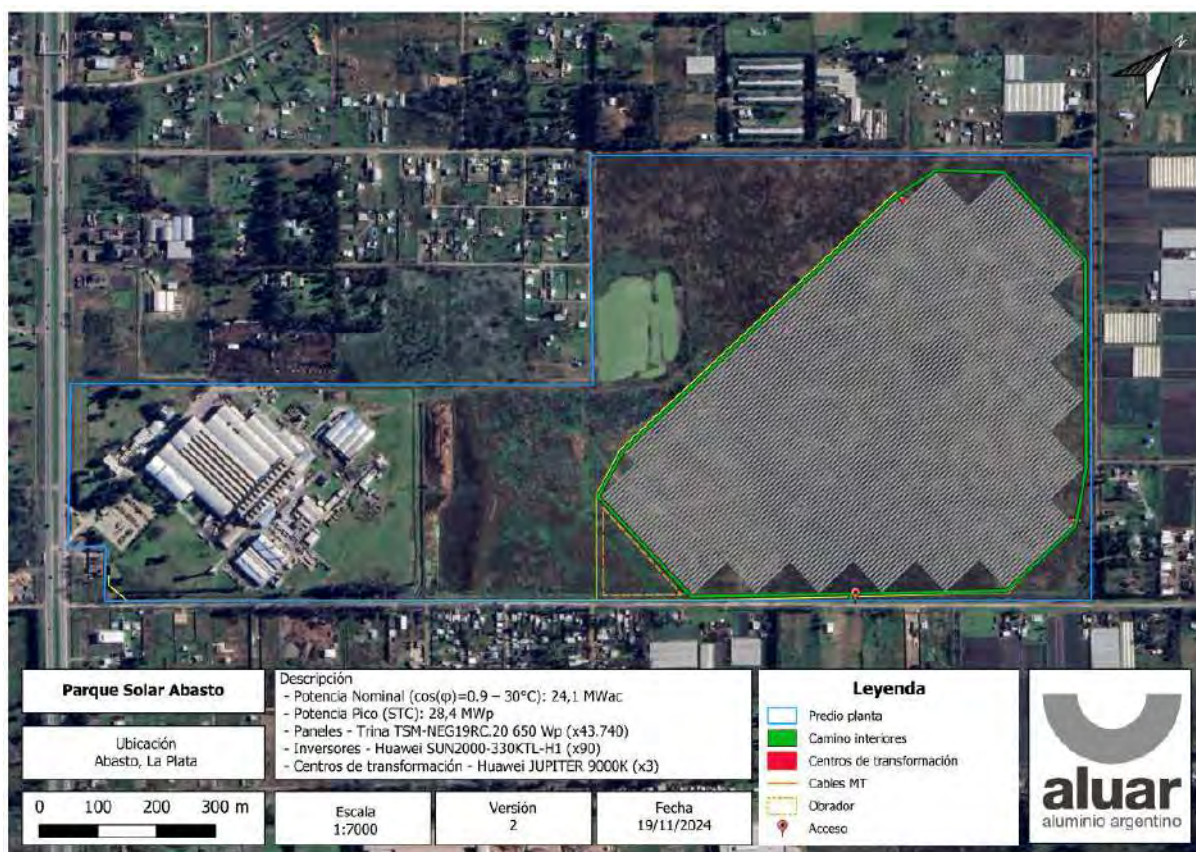
Figura 2.2-2. Layout del proyecto.
