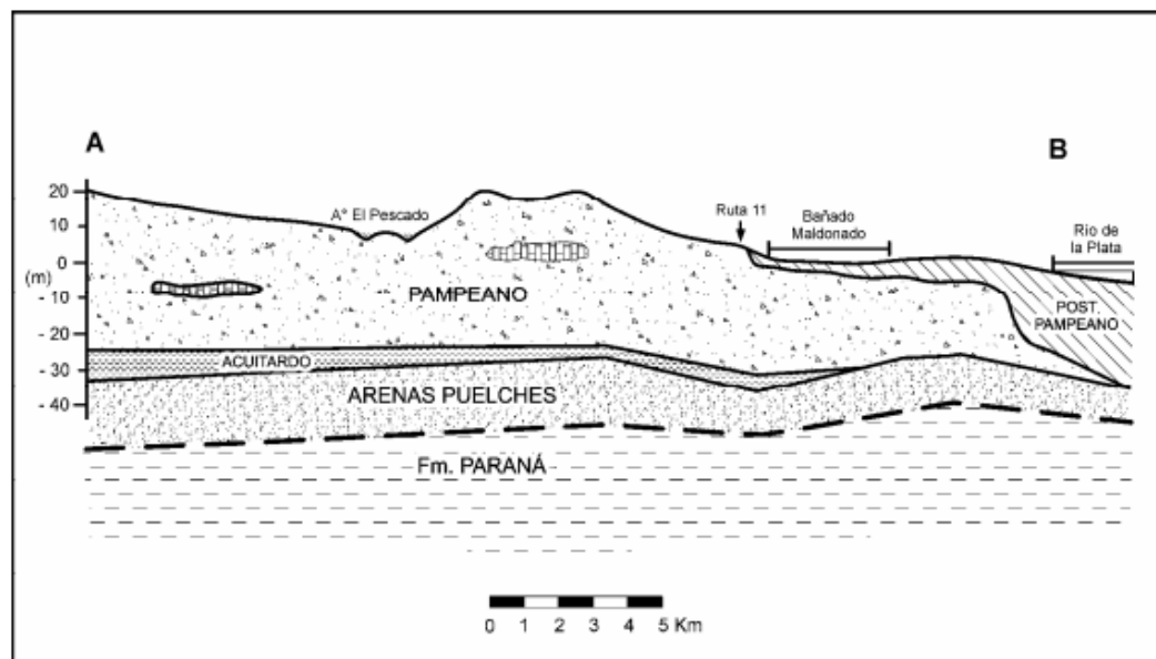
Figura 3.1-11. Perfil geológico.
