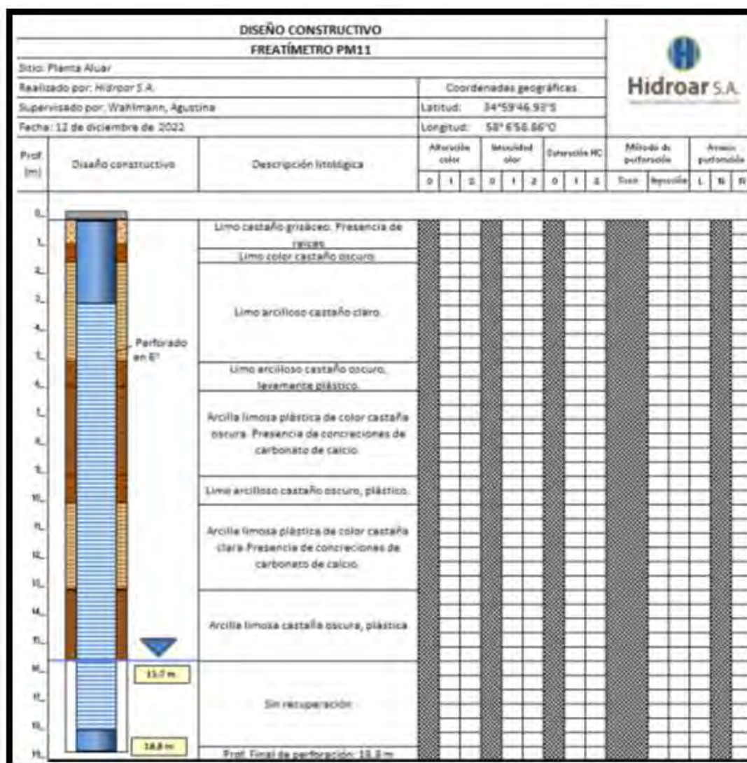
Figura 3.1-13. Freatímetros.
