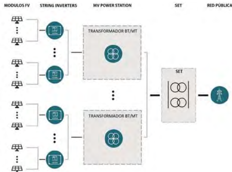
Figura 2.2-3. Esquema de configuración fotovoltaica del proyecto.
