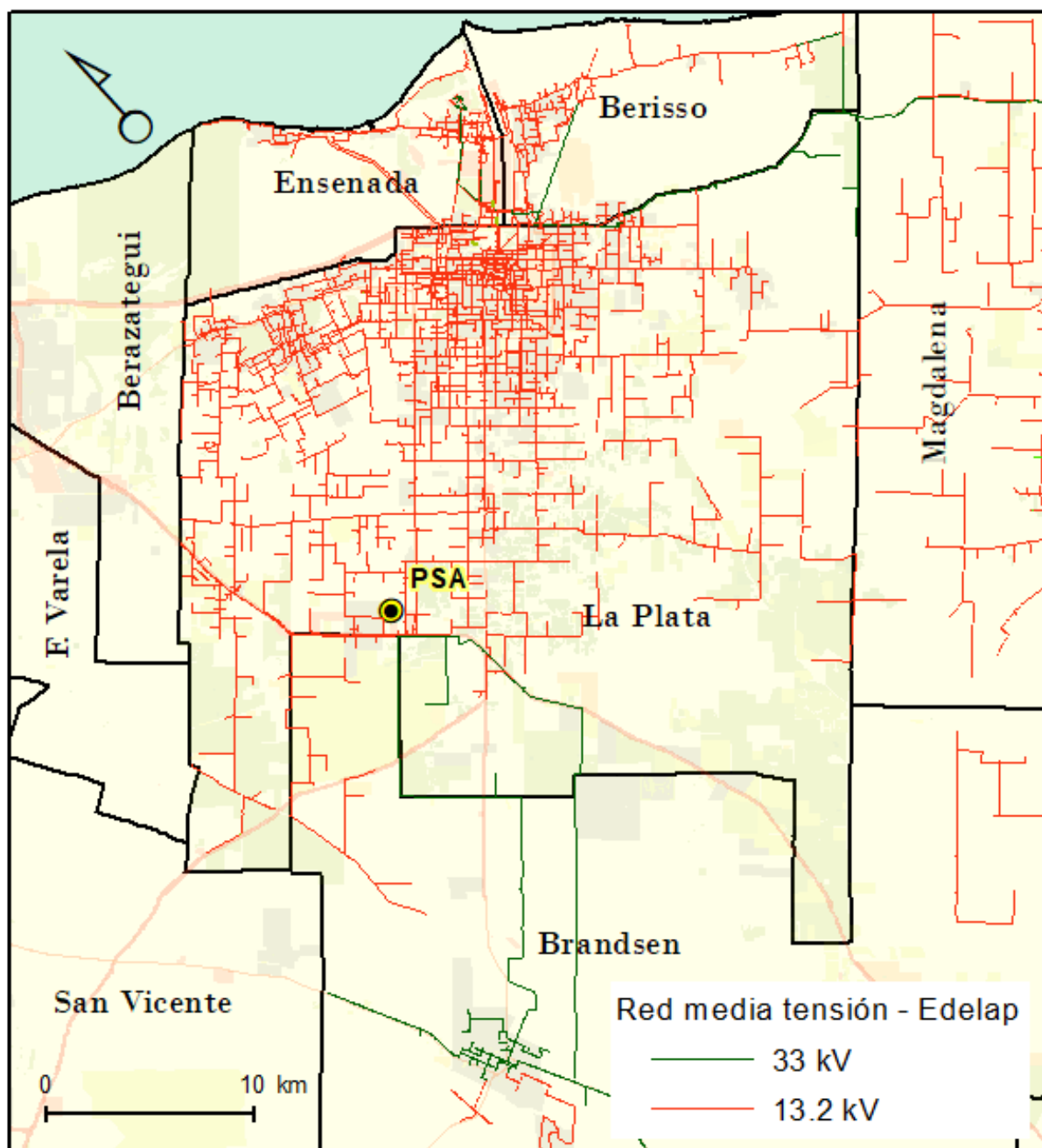
Figura 3.3-15. Mapa de la Red de Media Tensión – EDELAP. Fuente: Secretaría de Energía Argentina Nación. 2024.
