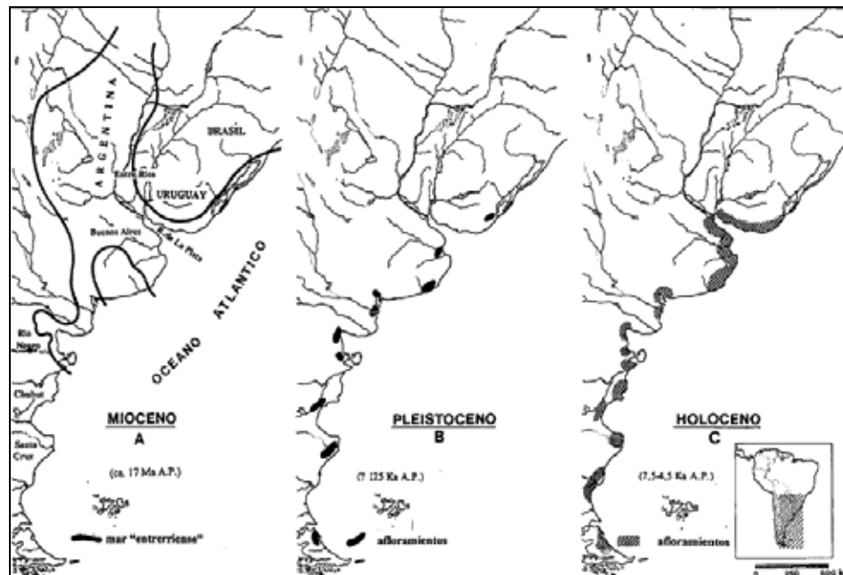
Figura 3.3-28. Transgresiones marinas a lo largo de la costa atlántica durante el Neógeno - Cuaternario. A: reconstrucción del área abarcada por el mar paranaense, B: detalle de los afloramientos pleistocenos, C: detalle de los afloramientos holocenos (Aguirre y Farinati, 1999).
